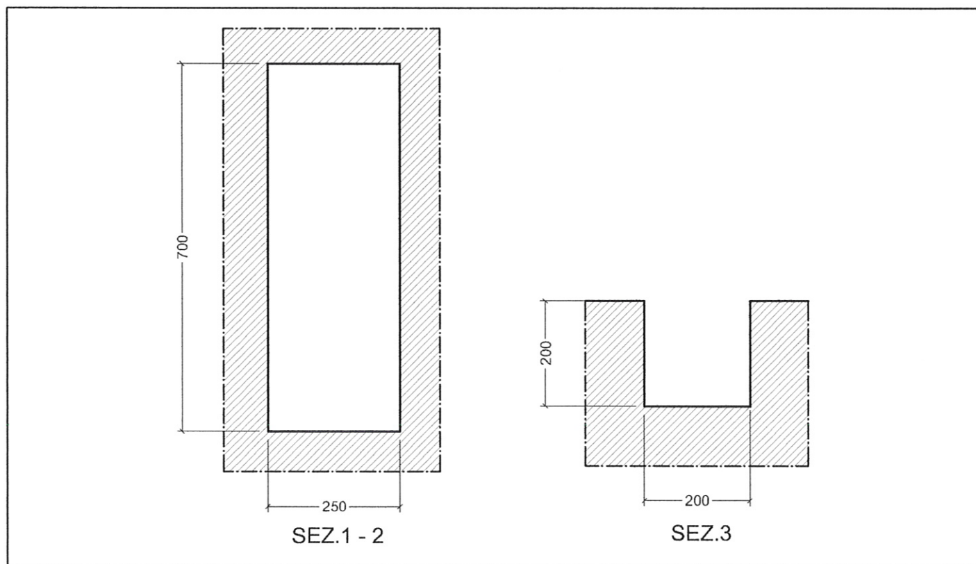
Sezioni scala 1:100
