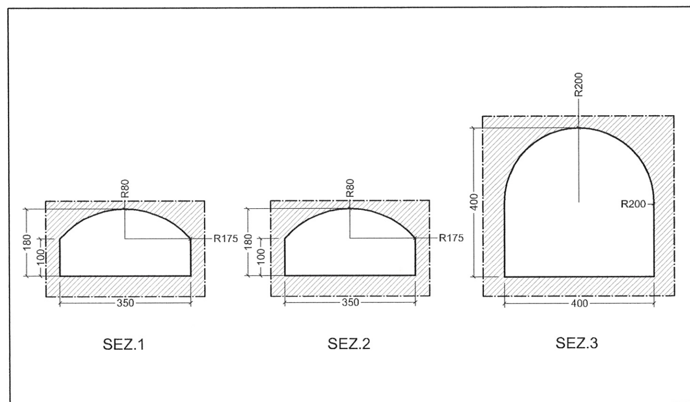
Sezioni scala 1:100
