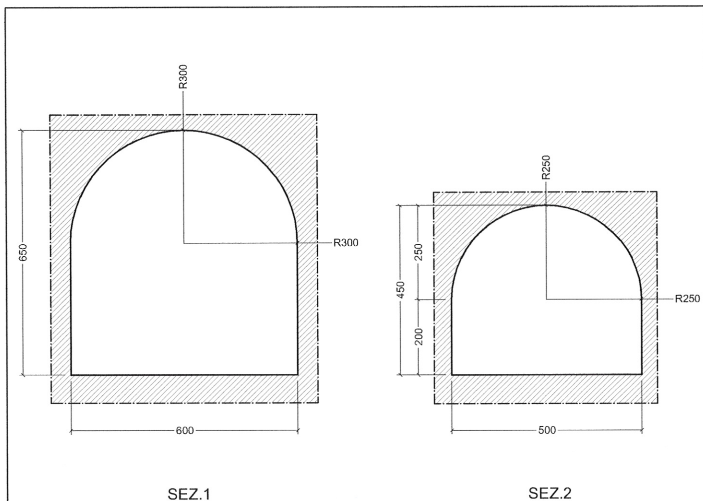
Sezioni scala 1:100
