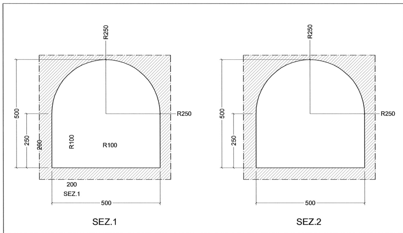
Sezioni scala 1:100
