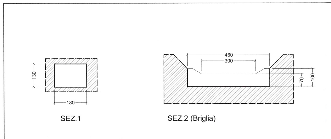
Sezioni scala 1:100
