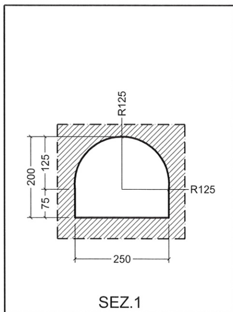
Sezioni scala 1:100
