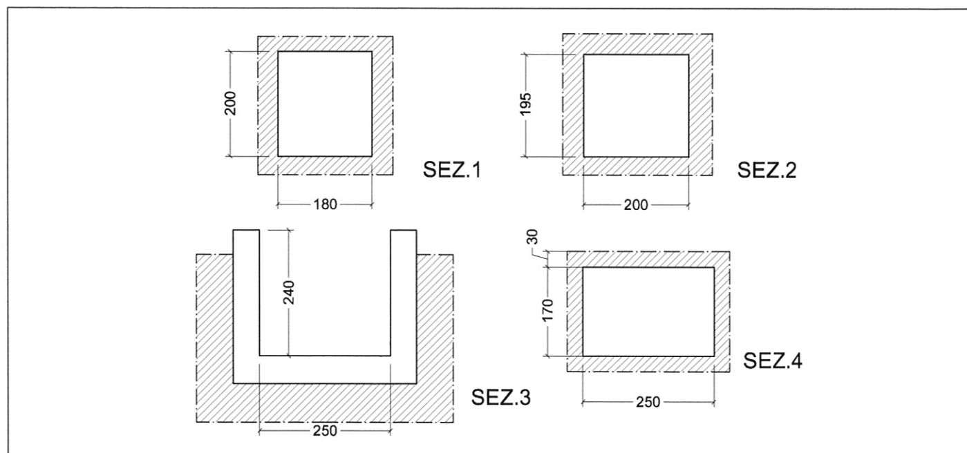
Sezioni scala 1:100
