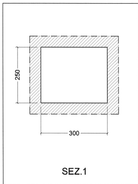
Sezioni scala 1:100
