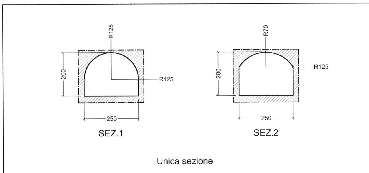
Sezioni scala 1:100
