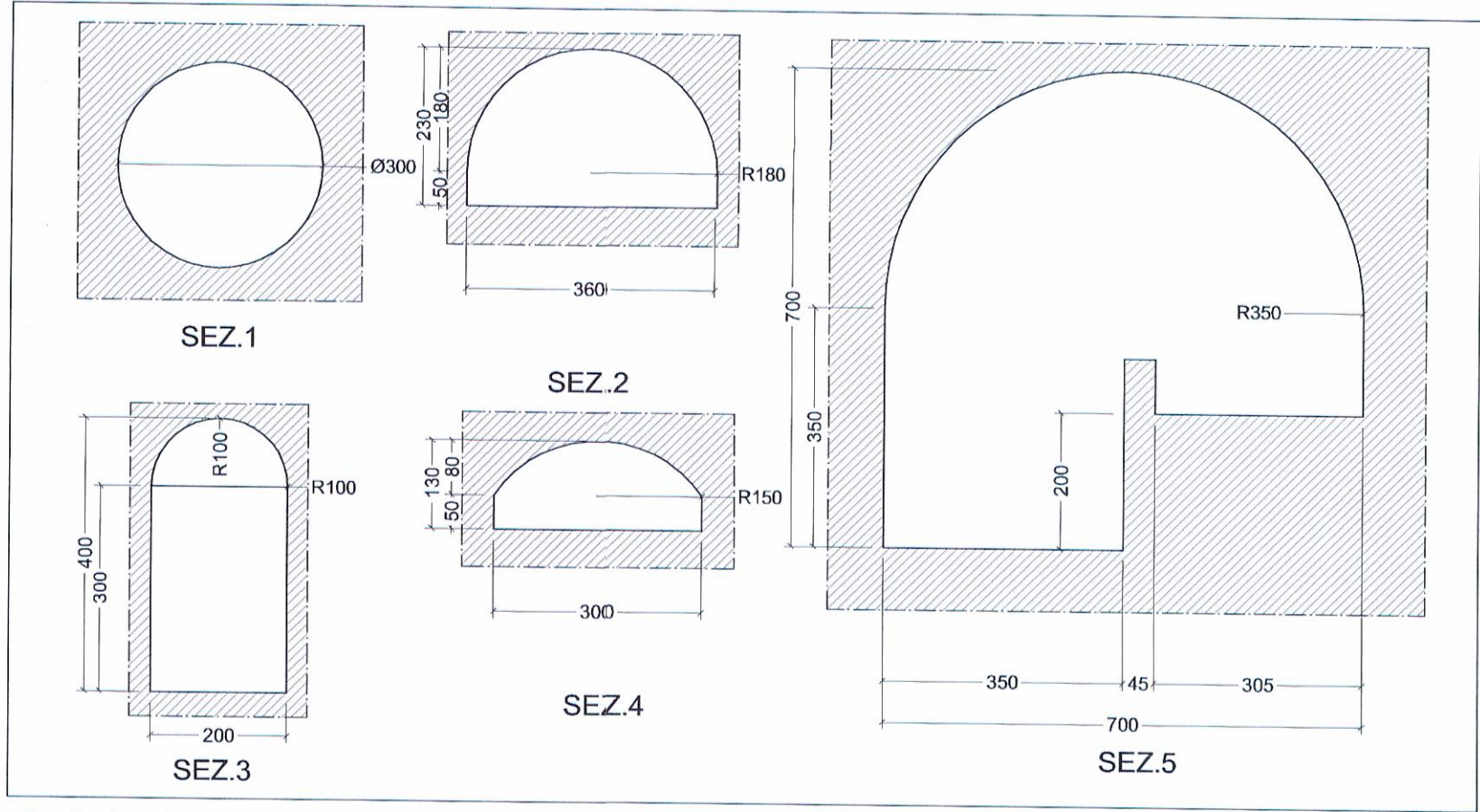
Sezioni scala 1:100
