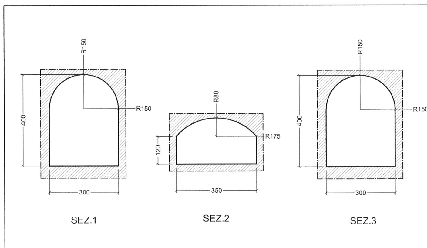
Sezioni scala 1:100
