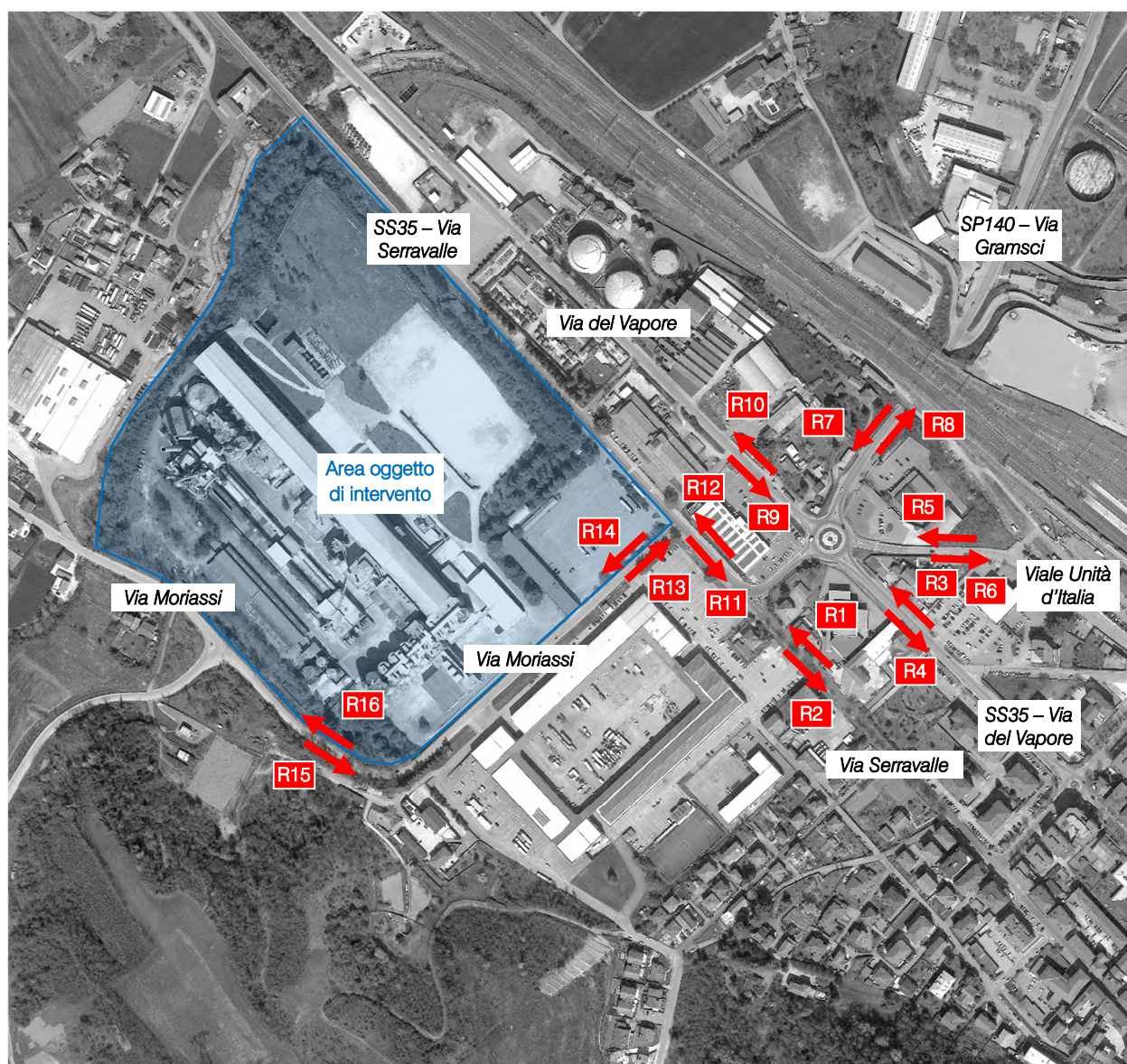
Figura B.1 – Sezioni di rilievo tramite strumentazione radar
