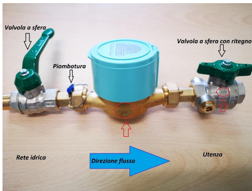
Figura 1: Allaccio standard
