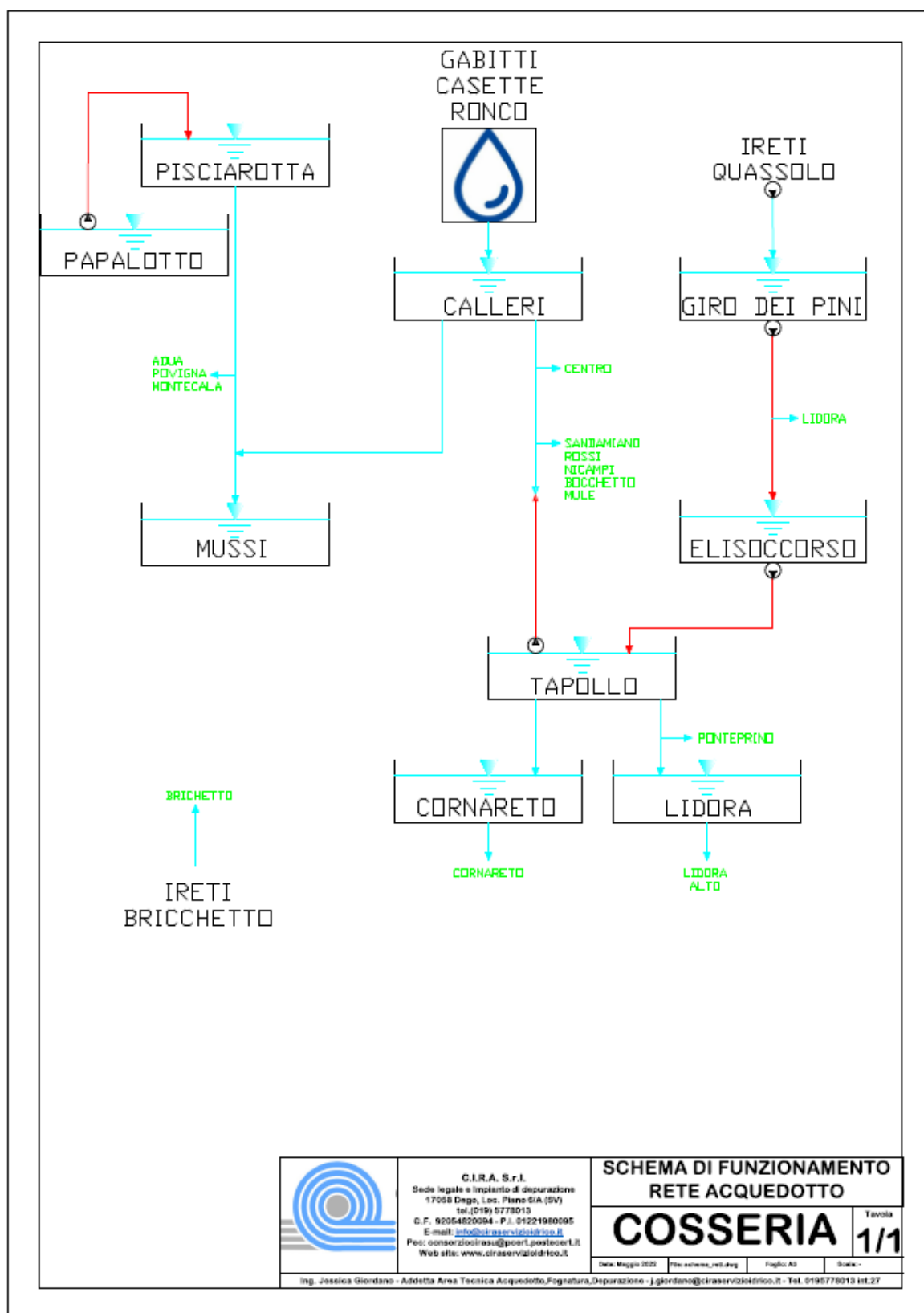
Figura 5: Schema funzionale rete comune di Cosseria stato attuale
