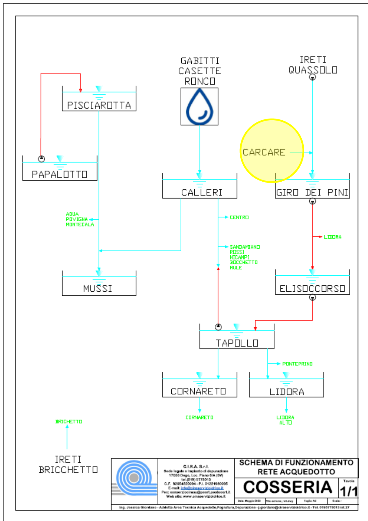
Figura 10: Schema funzionale rete comune di Cosseria in progetto
