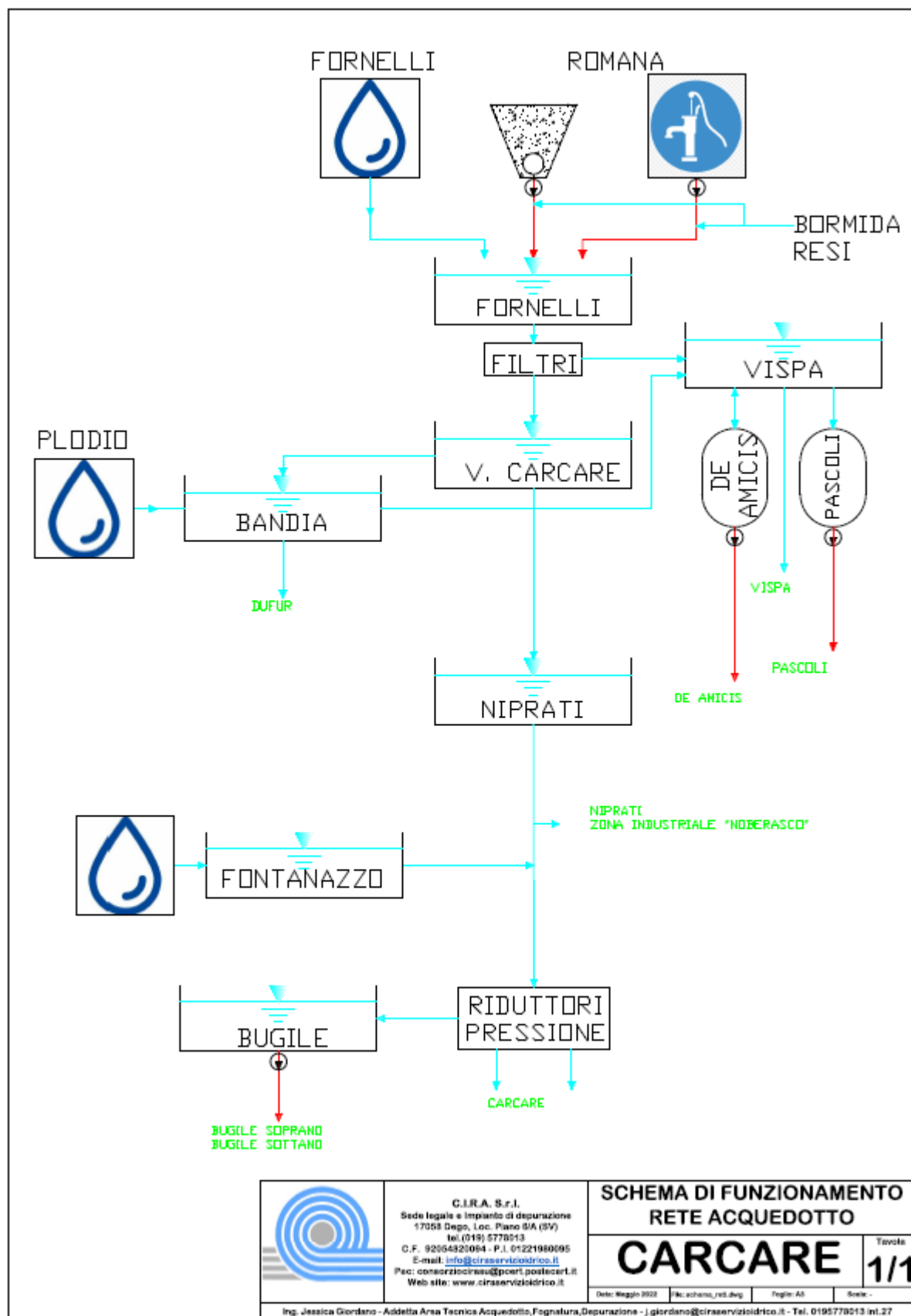
Figura 4: Schema funzionale rete comune di Carcare posto collegamento con rete Comune Bormida
