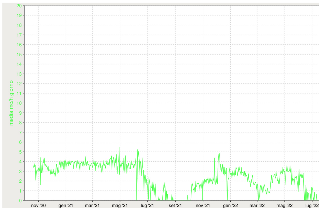
Figura 6: Portata in ingresso al serbatoio Tapollo – Alimentazione Calleri
