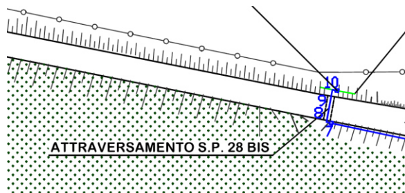
Interferenza n°4: Attraversamento S.P. 28 bis (tratto 7-10)
