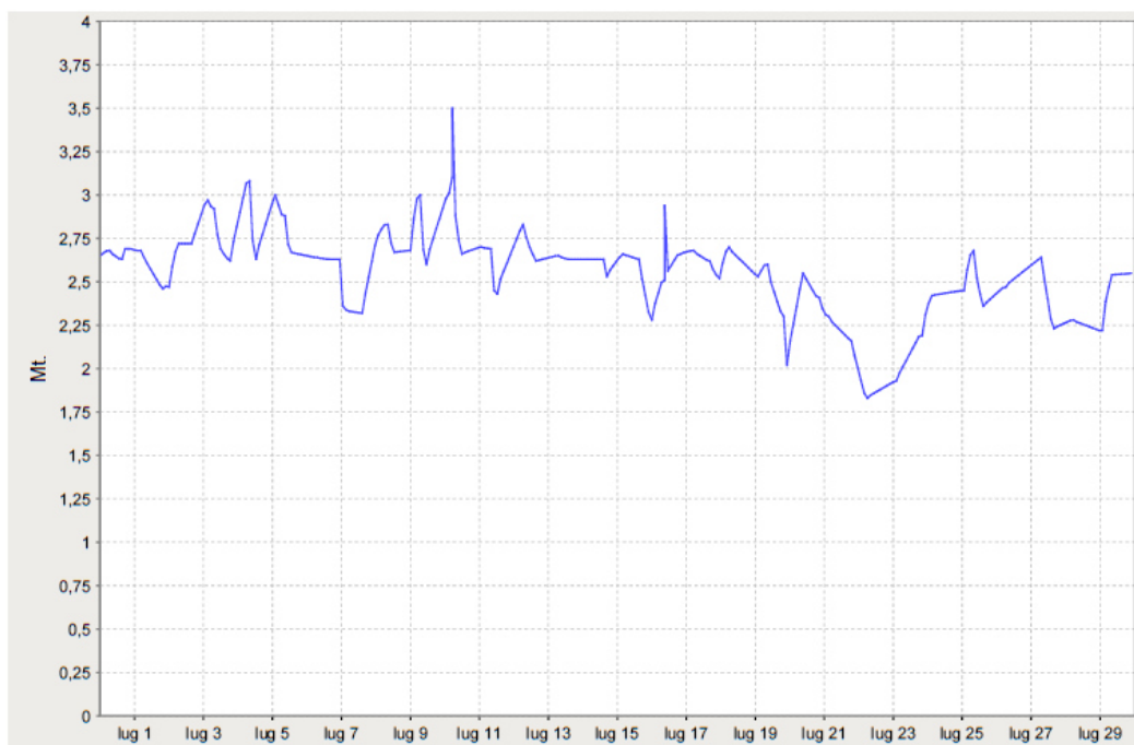
Figura 7: Livello serbatoio Calleri – Luglio 2021
