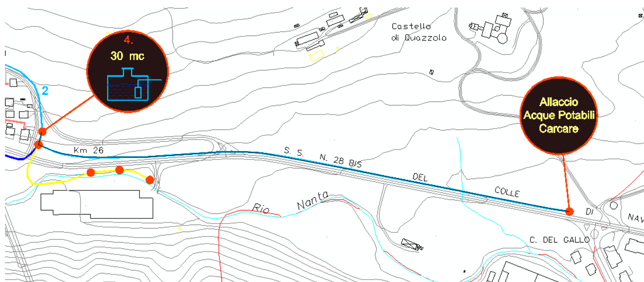
Figura 11: Tracciato di massima condotta esistente di collegamento Loc. Romana-Serbatoio "Fornelli"
