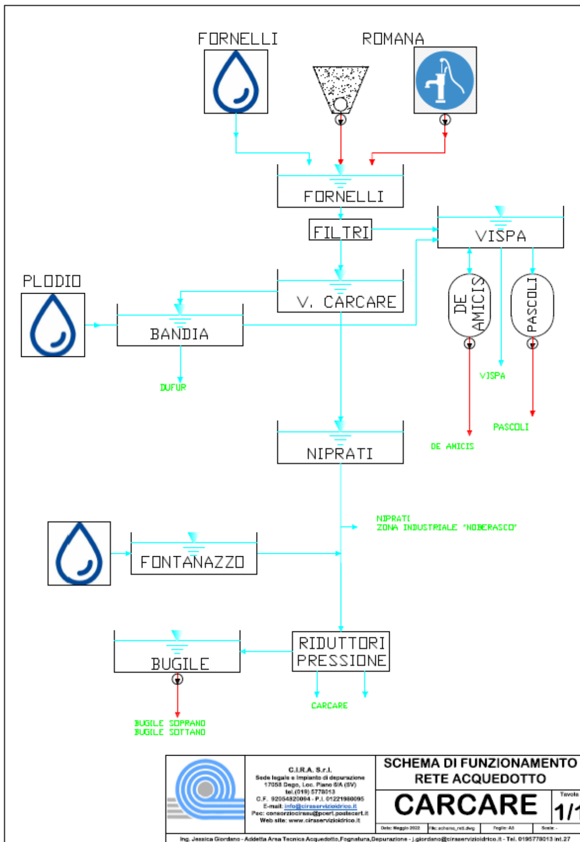
Figura 3: Schema funzionale rete comune di Carcare stato attuale
