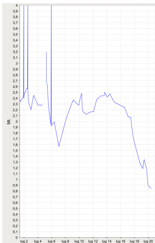
Figura 8: Livello serbatoio Calleri – Luglio 2022
