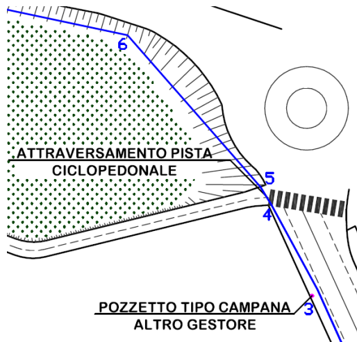
Interferenza n°2: Parallelismo condotta altro gestore e allacci (tratto 3-6)
