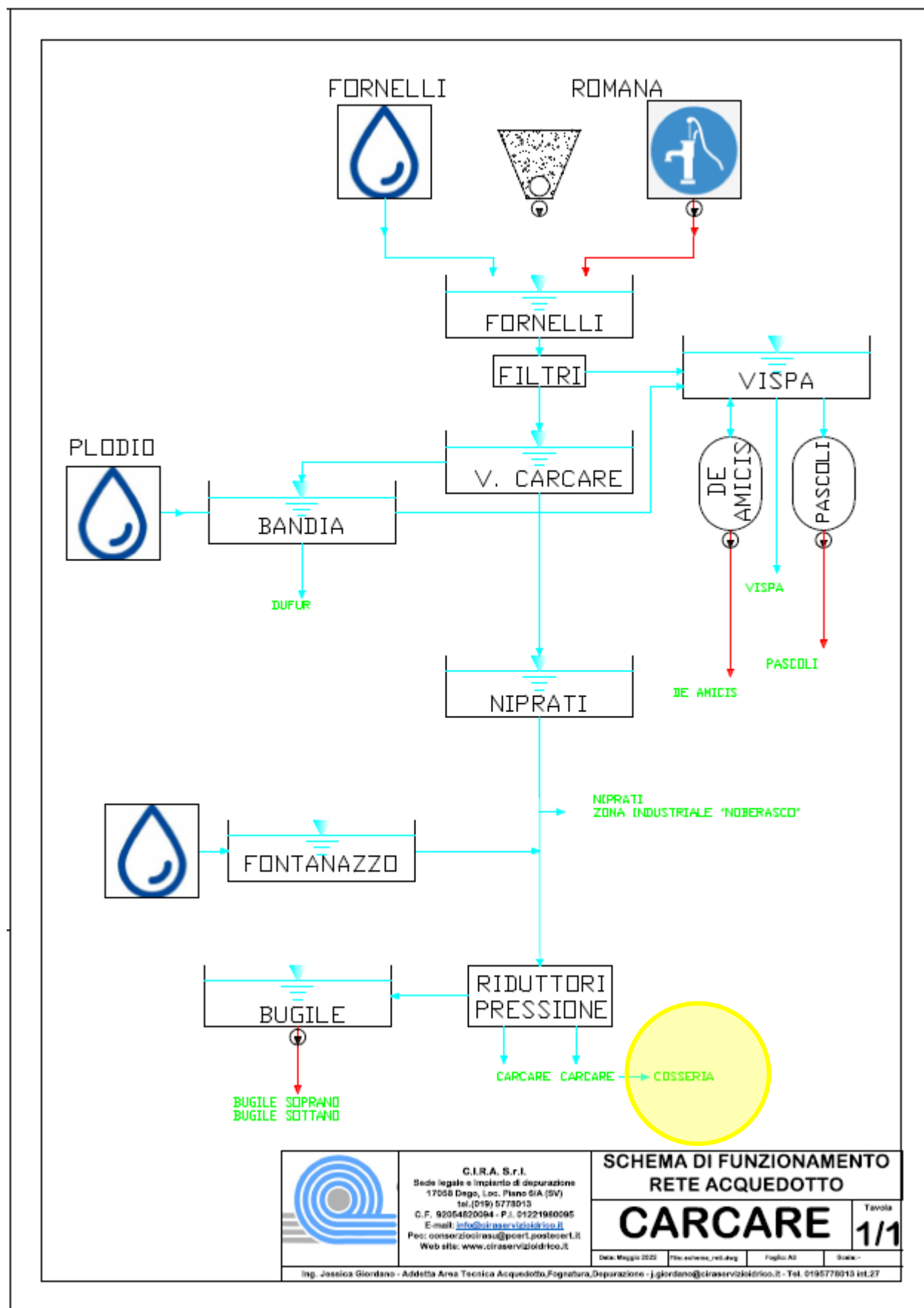
Figura 9: Schema funzionale rete comune di Carcare in progetto
